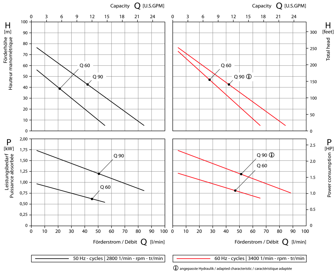
Abbildung: Neue Kennlinien CY-4281-MK, TOE/CY-4281-MK und Y-4081
